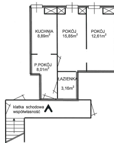
UPROSZCZONY SZKIC LOKALU MIESZKALNEGO NR 9 BOLESŁAWIEC ul. Rynek 29/30 podłoga 2 piętra działka nr 271, IX obręb ewidencyjny instalacje: elektryczna, wodna, kanalizacyjna, gazowa wysokość pomieszczeń - powyżej 2,50m; powierzchnia użytkowa - 48,52m 2
