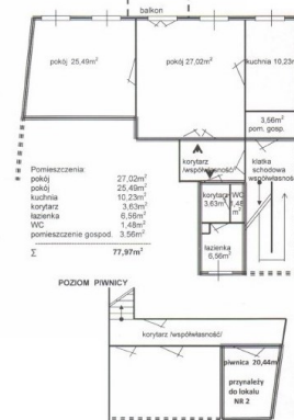
UPROSZCZONY SZKIC LOKALU MIESZKALNEGO NR 2 BOLESŁAWIEC ul. Kutuzowa 11 początek 1 piętra Instalacje elektryczna, wodna, kanalizacyjna, gazowa wysokość pomieszczeń - powyżej 2,50m powierzchnia użytkowa - 77,97m 2
