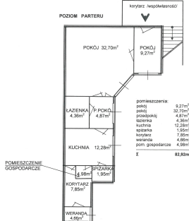
UPROSZCZONY SZKIC LOKALU MIESZKALNEGO NR 1 89-708 Bolesławiec, ul. Komuny Partyjskiej 8 działka nr 59/7, etery IX
